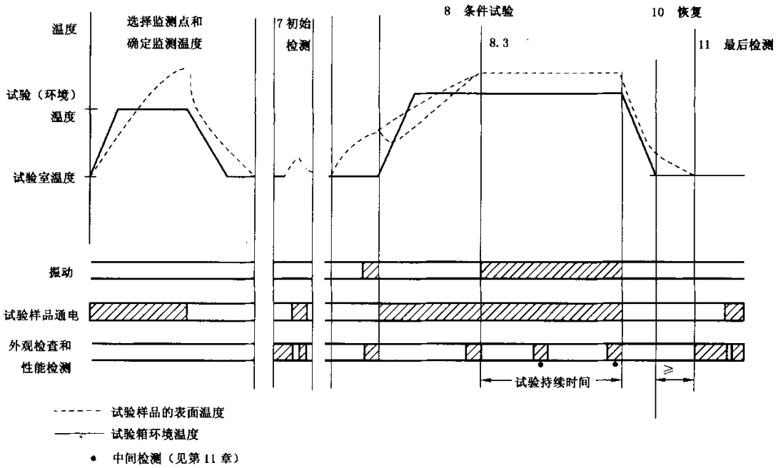
图2 散热试验样品试验曲线图
